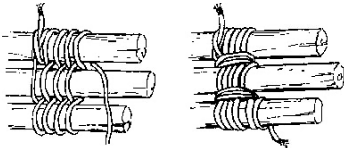
Stap 2. De palen aan elkaar weven. Let op: op de afbeelding zijn er slechts 3 palen gebruikt. Voor de decoratietrap gebruik je er 4, maar de techniek blijft hetzelfde.
